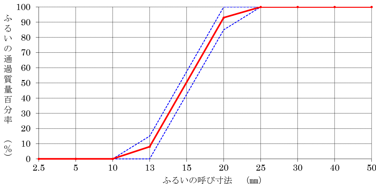
粒度曲線図
